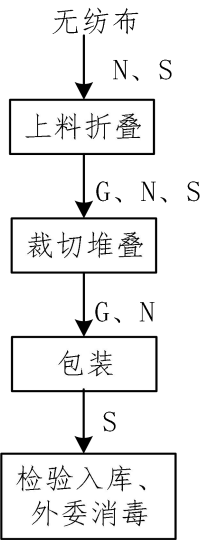
图 2-3 医用棉片生产工艺流程及排污节点图
